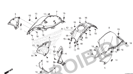
C-22 Carenagem (CG160ED/EDC/EDP)
