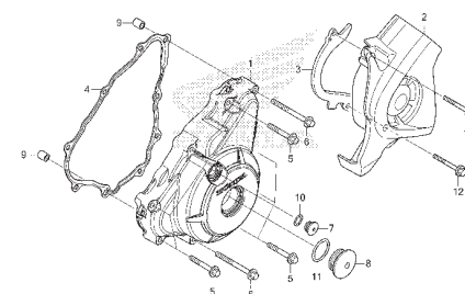
M-10 Tampa Lateral Esquerda
