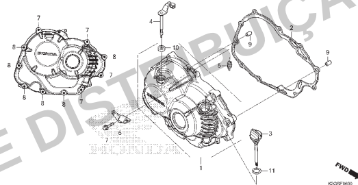
M-10 Tampa Lateral Esquerda
