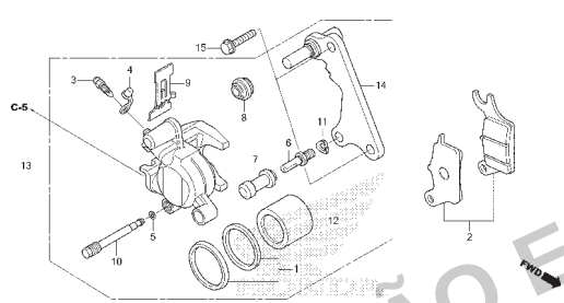
C-12 Cáliper do Freio Dianteiro (CG160ED/EDC/EDF/EDP)
