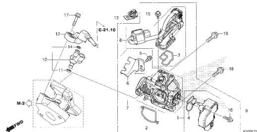
M-23 Corpo do Acelerador • Injetor de Combustível
