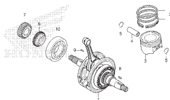
M-16 Árvore de Manivelas • Pistão
